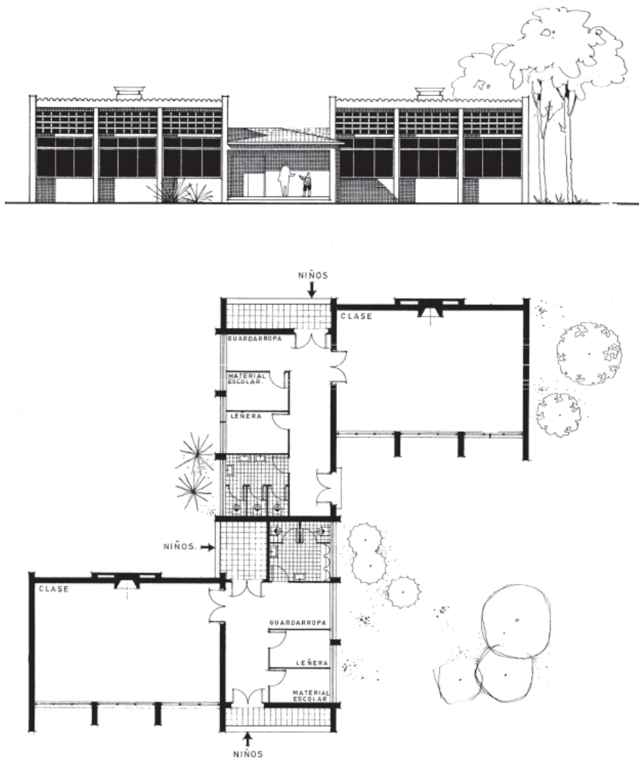
14 Esquema modular de escuelas usado por José Luis Fernández del Amo Moreno en El Trobal (Sevilla), 1962; y por Jesús Ayuso Tejerizo en Nuevos Francos (Salamanca), 1963
