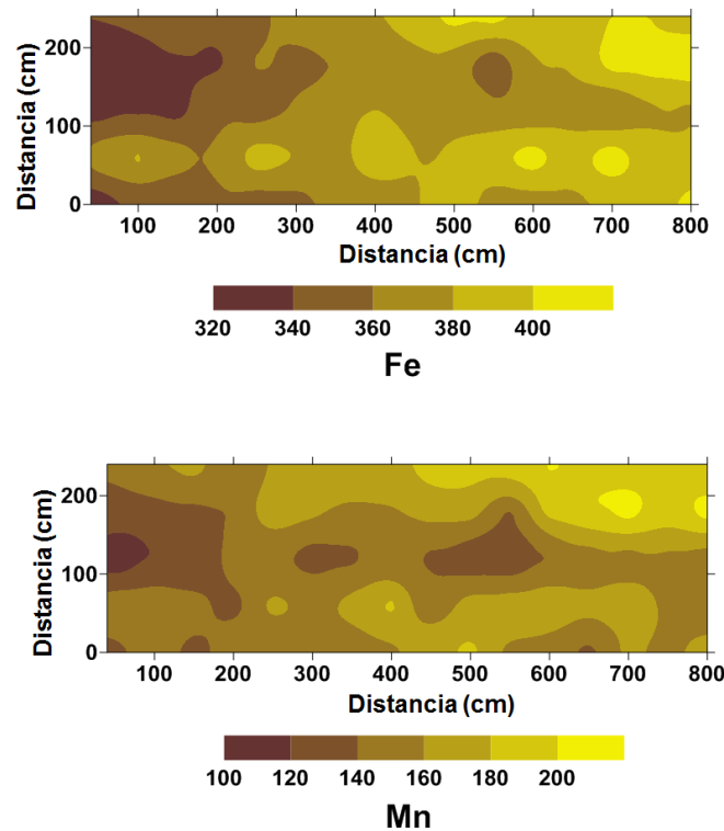
Figura 3. Mapas de krigado para Fe y Mn en la microparcela (mg/kg).
